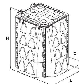
Horto 200/300/400 forma conico-trapezoidale
